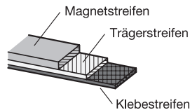
Magnetband
